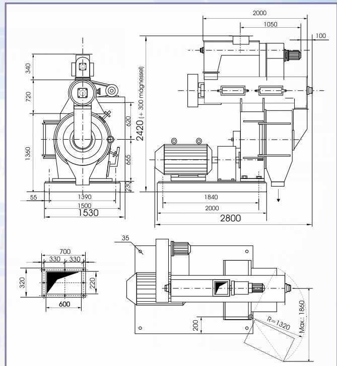
Gránit-132 granulálógép rajza / Outline drawing of the Gránit-132 pellet mill
