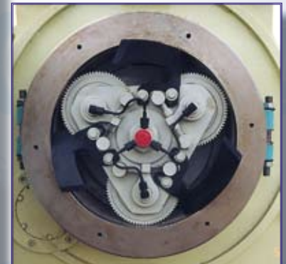
Présgörgők, matrica a Gránit-90-es granuláló gép munkaterében / Pellet die and pellet rolls of Gránit-90 pellet mill
