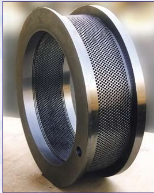
Gránit-90-es présma- trica / Pellet die for Grá- nit-90 pellet mill
