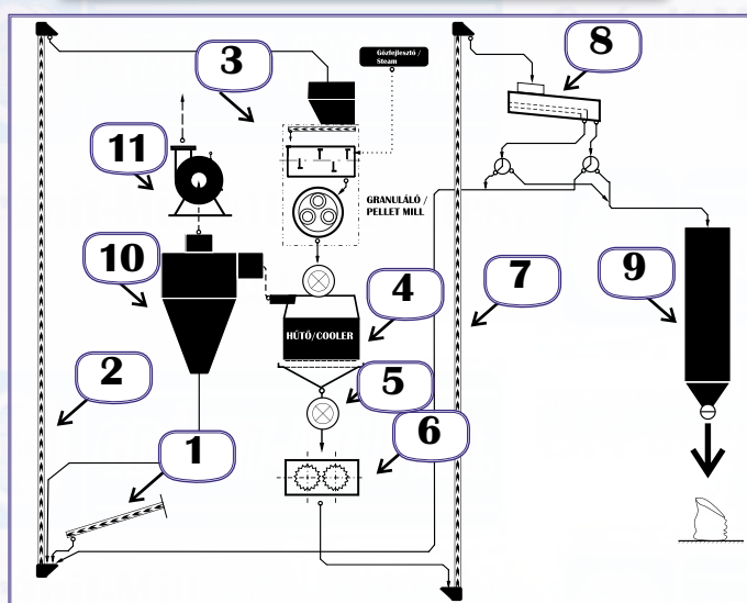
Az egyes gépek helye a préstechnológiában / Machines' location of the pellet producing line
